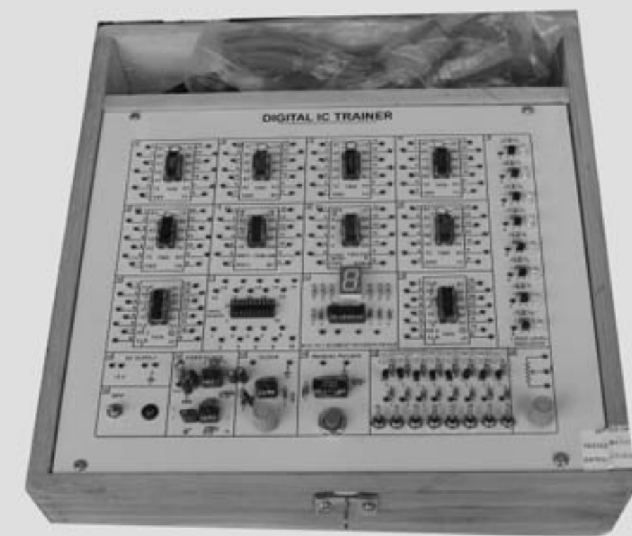
Digital I C Trainer
